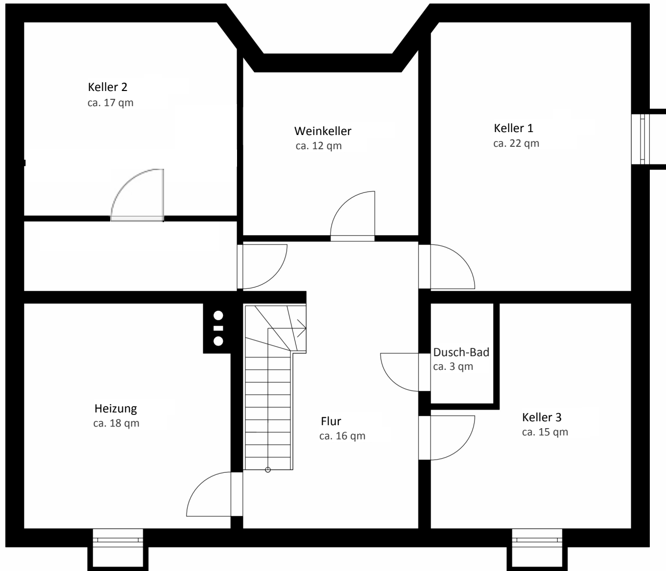
Kellergeschoss
